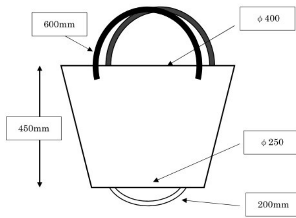
(2) 小型タイプ
