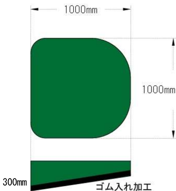
(1) 大型車用ゴム入りホッパーカバー
