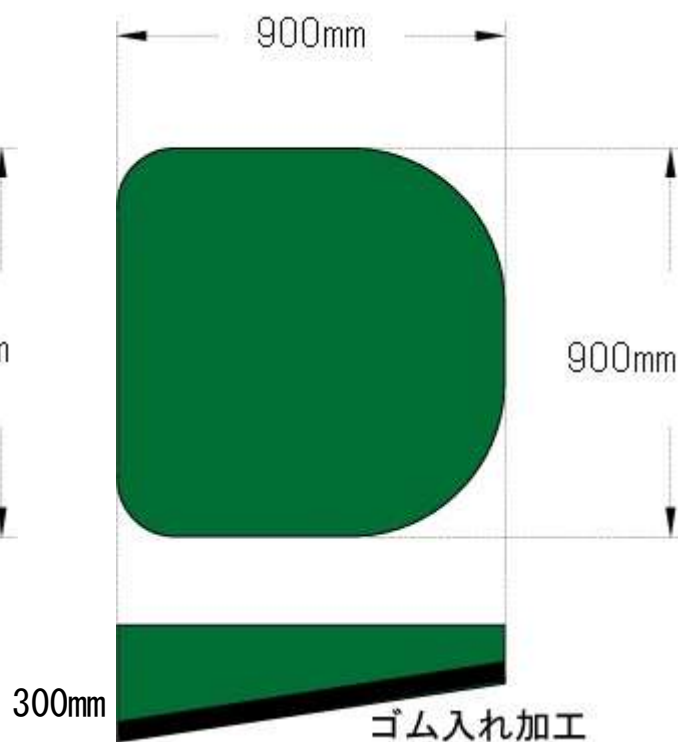
(2) 小型車用ゴム入りホッパーカバー
